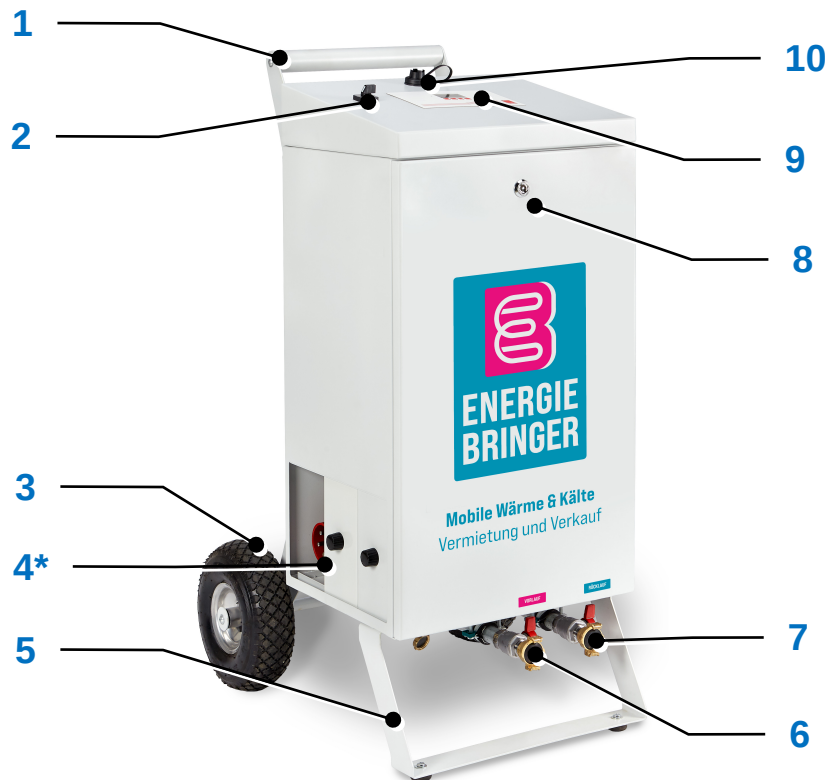
Abb. 1): Außenansicht der mobilen Heizzentrale (beispielhaft)
