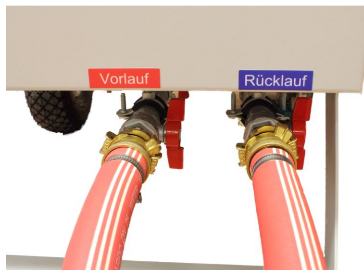
Abb. 8): Verbindungsschläuche DN25 am Heizungsvor- und -rücklauf der mobilen Elektroheizzentrale - Armaturen sind geschlossen -
