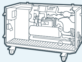
FRISCHWASSERMODUL 140 kW
