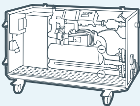
FRISCHWASSERMODUL 60 kW
