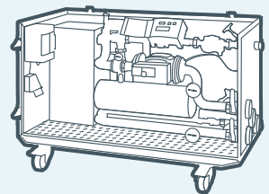
FRISCHWASSERMODUL 502 kW
